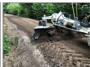
Abgerandete Flurstrasse / bestehendes Kies profilieren
